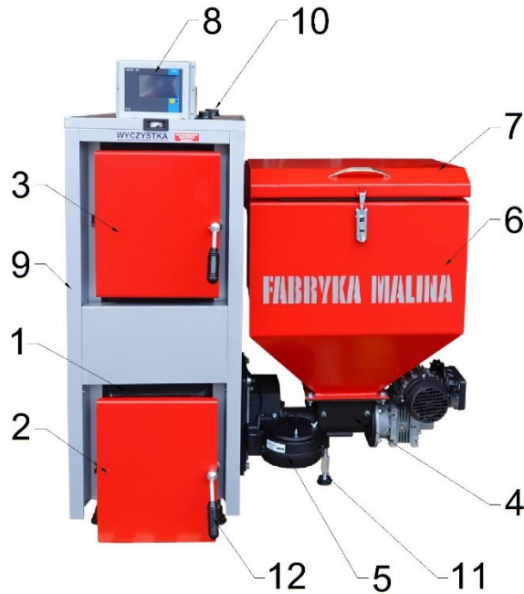
Rys.2. Kocioł „MALINA PREMIUM”
